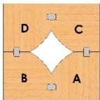
KUVA. Periaatepiirrokset neliöontelopilarista
