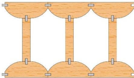
KUVA. Periaatepiirros seinä- & välipohjaonteloelementistä.
