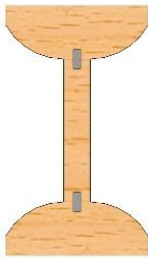
KUVA. Periaatepiirros pienpalkista.
